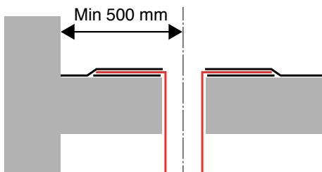
Takbrunnar och bräddavlopp ska placeras minst 500 mm från vertikal yta (vägg, sarg o.d.). Detta för att anslutning av tätskikt mot hel fläns ska vara möjlig. Fläns till takbrunn och bräddavlopp får aldrig klippas eller vikas.
