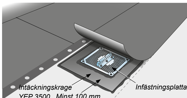
Alternativ 1. Tätskiktet helsvetsas mot infästningsplatta och intäckningskrage av YEP 3500.
