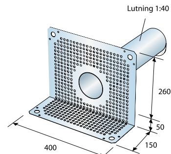
Sargbräddavlopp
