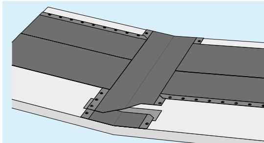
Rännalsvåd alternativ 1 – förstärkningsremsa YEP 3500 under tvärskarv
