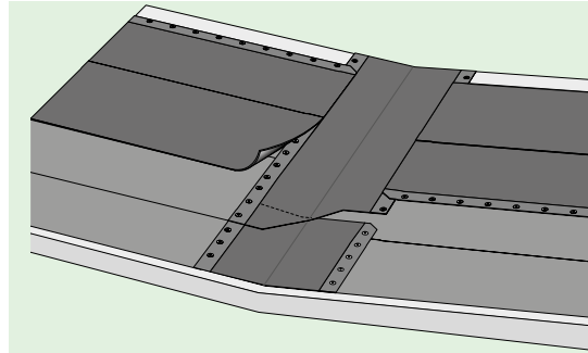
Rännalsvåd alternativ 1 – förstärkningsremsa YEP 3500 under tvärskarv
