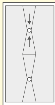
C. Motfallstak med rännalskilar. (fall mot takbrunnar i ränn dalen) Takbrunnar kan inte samverka – det krävs ett bräddavlopp per takbrunn.
