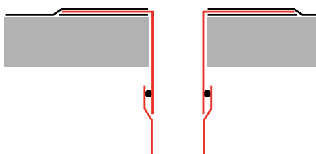
Tappestycke till brunn och bräddavlopp ska ha en sådan längd att anslutning till stuprör utförs under tak- eller bjälklagskonstruktion.
