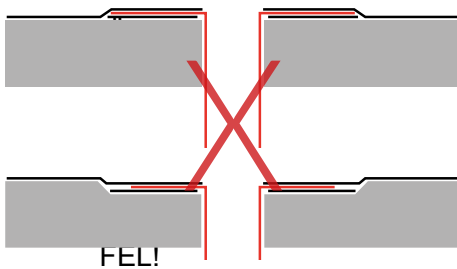
Takbrunnar och bräddavlopp ska inte försänkas i underlaget.
