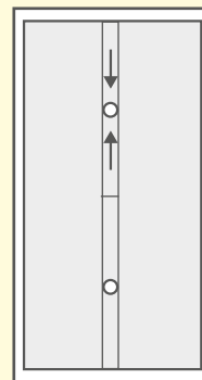
D. Motfallstak med lutande försänkt ränn dal. Takbrunnar kan inte samverka – det krävs ett bräddavlopp per takbrunn.
