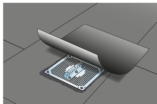
Alternativ 2. Tätskiktet helsvetsas mot infästningsplatta och tätskiktsmatta. Storlek på tätskiktsbit över infästningsplatta ska vara enligt anvisning från leverantör av aktuell infästningsplatta. Tätskiktsbiten ska dock nå minst 150 mm utanför plattan på alla sidor.
