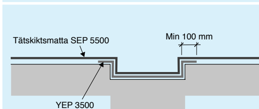
Försänkt rännal Vid försänkt rännal ska tättskiktet utföras som 2-lagstäckning i hela rännaldalen.
