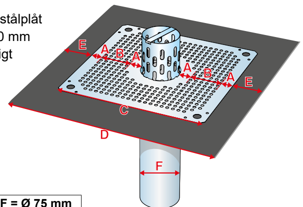
Brunn med perforerad rostfri fläns.
