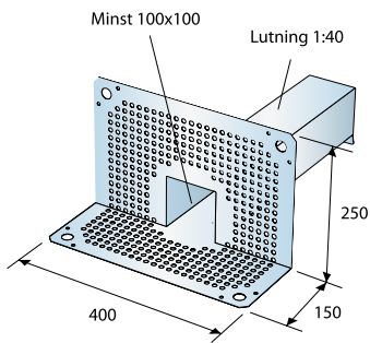
Utkastare
