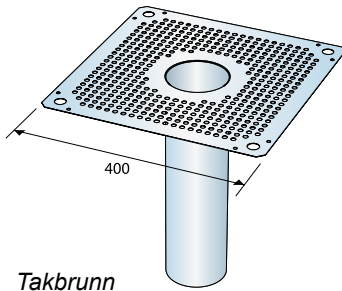
Takbrunn
