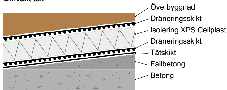
Omvänt tak
