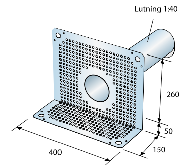
Sargbräddavlopp
