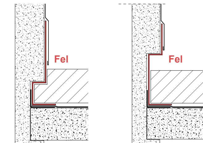
Utrymme byggs igen så att tätskiktet kan dras rakt upp.
