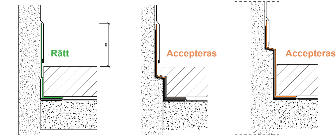
Uppvik ska utföras med dubbla tätskikt.
