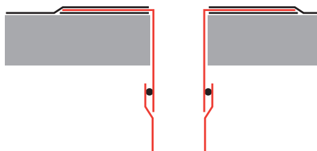
Tapstycke till brunn och bräddavlopp ska ha en sådan längd att anslutning till stuprör utförs under tak- eller bjälklagskonstruktion.
