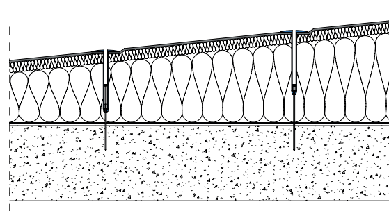
Fallupbyggnad i fallisolering
